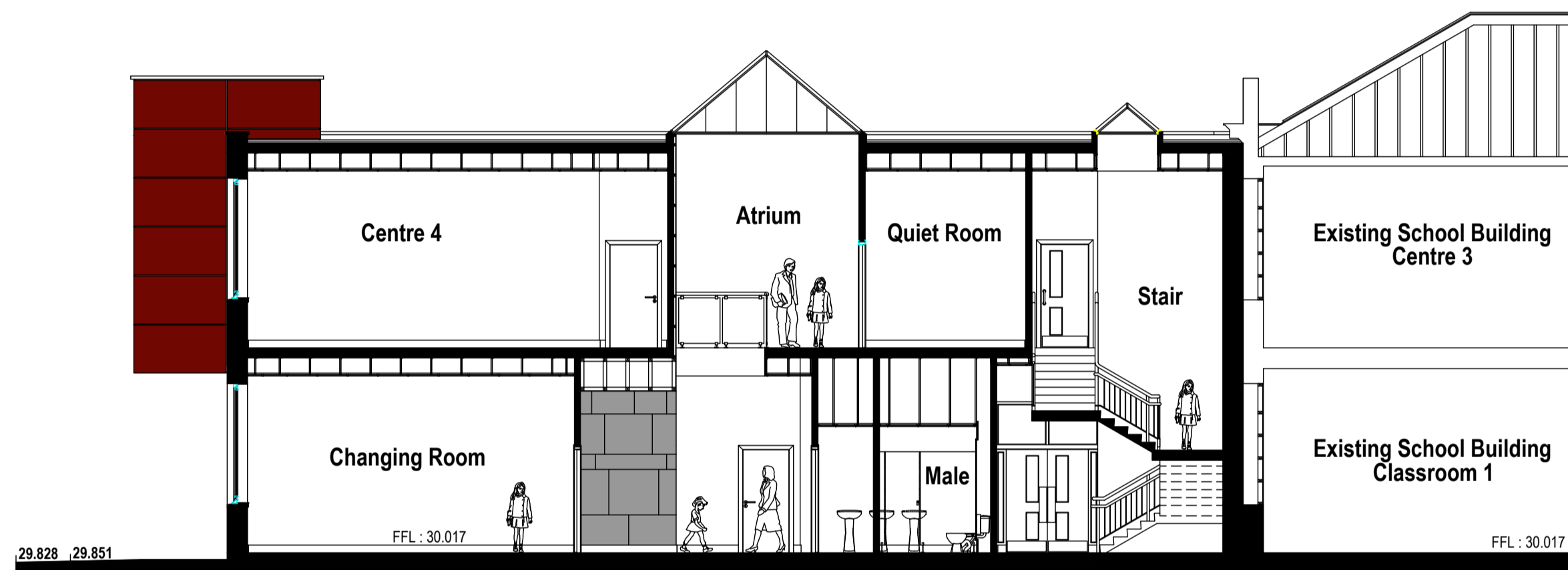
CROSS - SECTION E - E
